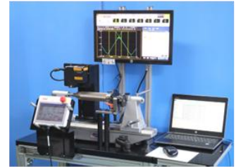
セレーション測定装置写真
